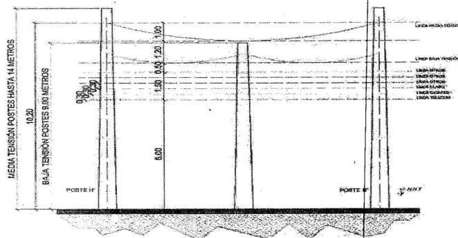
VISTA ESCALA: 1:100
