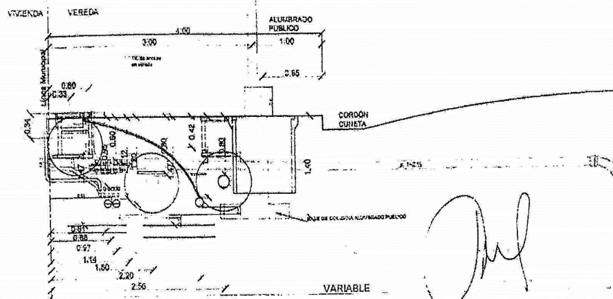
CORTE TRANSVERSAL DE DISTRIBUCIÓN DE REDES DE INFRAESTRUCTURA
