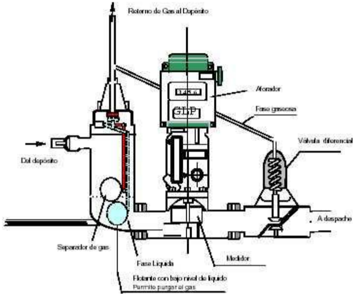
Figura 4: ESQUEMA TÍPICO DE SEPARADOR DE FASE GASEOSA
