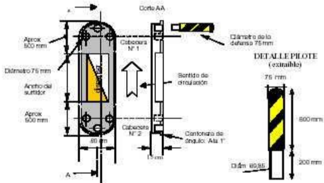
Figura N° 6: Tipo de ubicación en estación de carga cautiva
