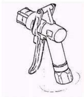
Figura 3 b: ESQUEMA BASICO DEL PICO DEL DISPENSER PARA G.L.P.A.
