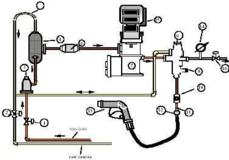
Figura 3: Esquema básico de un dispenser de G.L.P.A.
